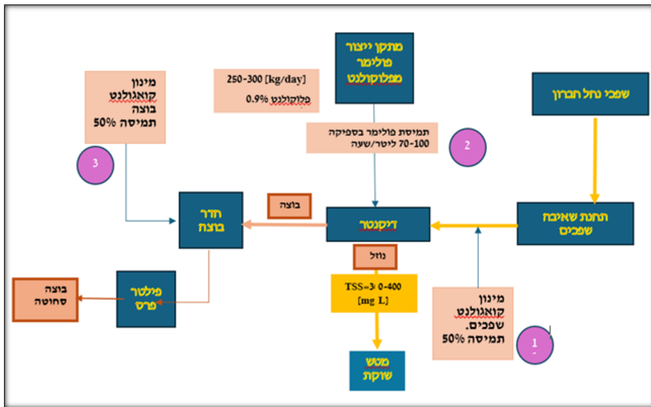
איור 1- מערכת מינון כימיקלים במתקן תפיסה חברון
